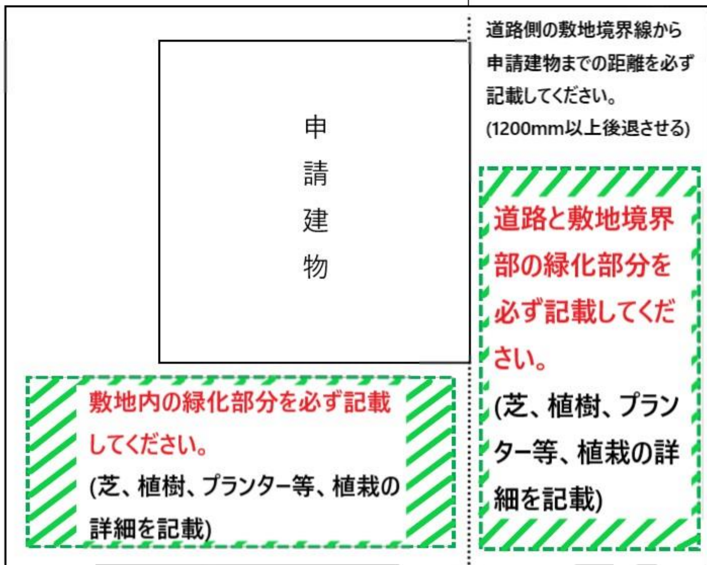
配置図
