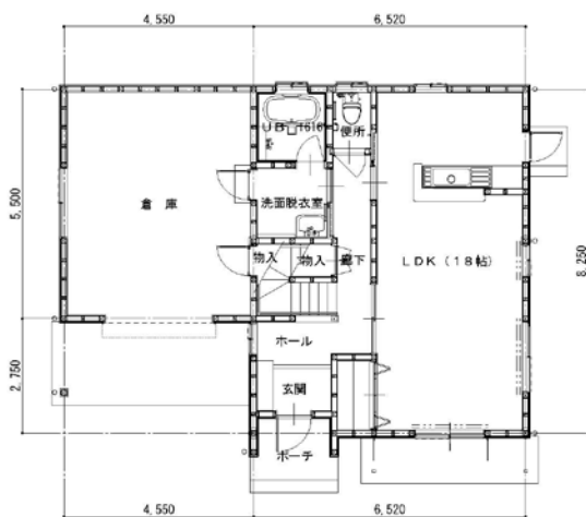
1階 平面図
