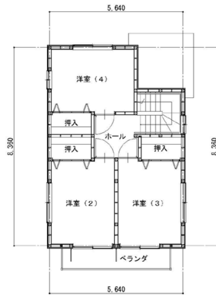
2階 平面図
